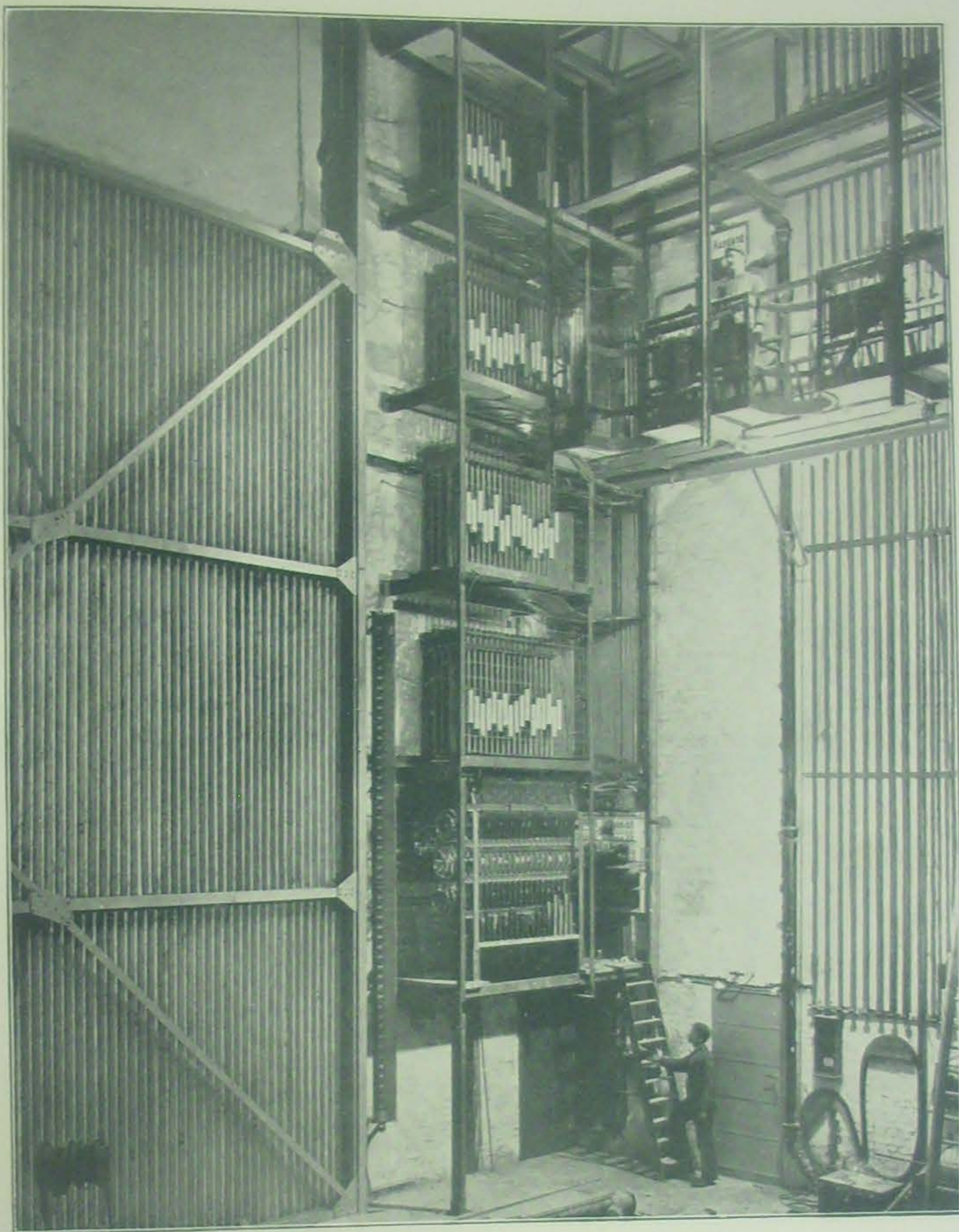
Bühnenregulator, Komische Oper · Berlin.
