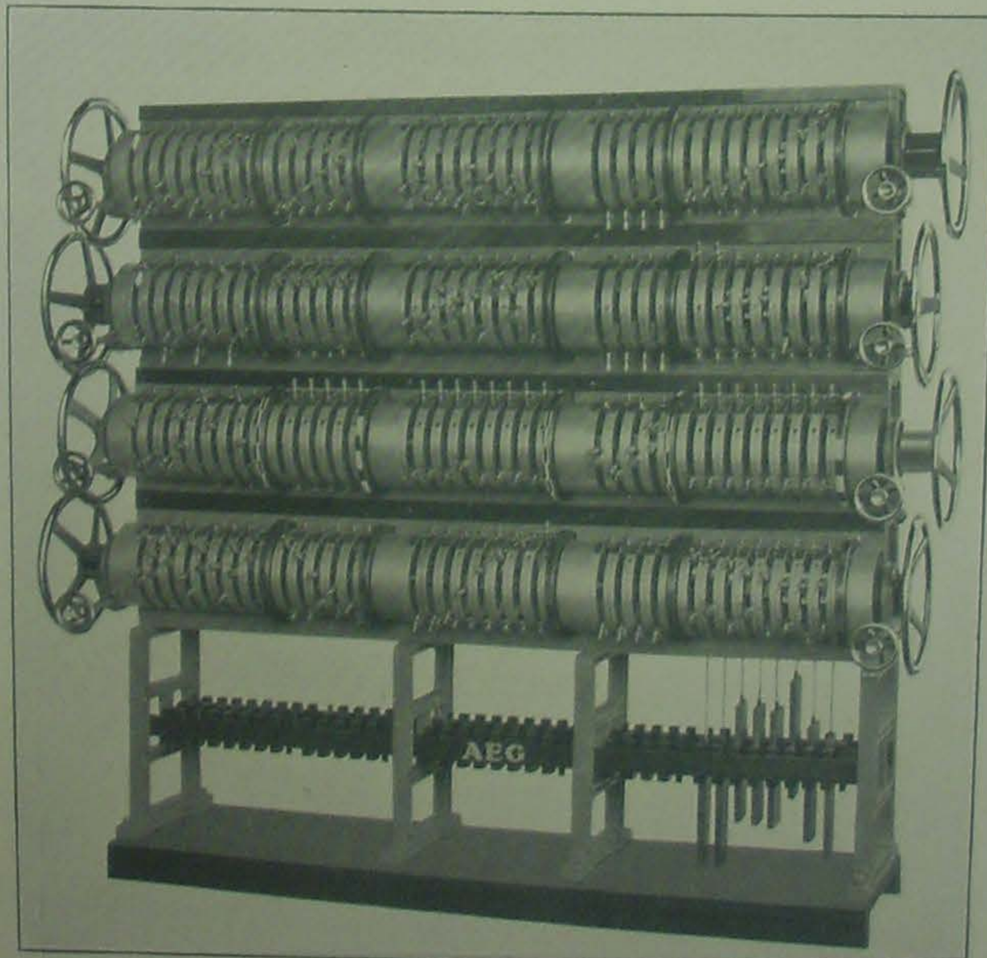
Stellwerk des Bühnenregulators mit 4 \times 33 Hebeln.
